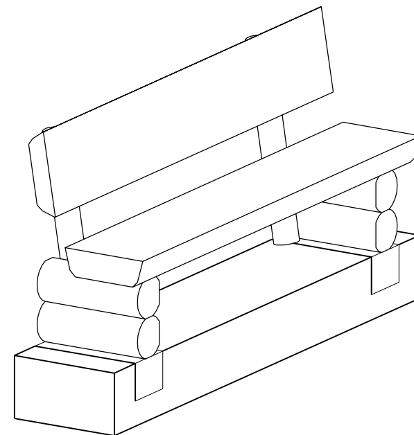
VISTA AXONOMÉTRICA Escala: 1:20
