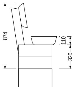
VISTA EN PERFIL Escala: 1:30
