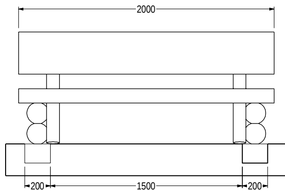
VISTA EN ALZADO Escala: 1:30
