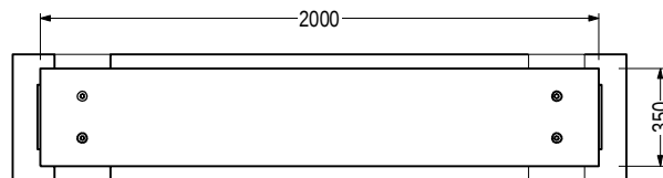
VISTA EN PLANTA Escala: 1:30
