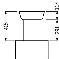
VISTA EN PERFIL Escala: 1:30
