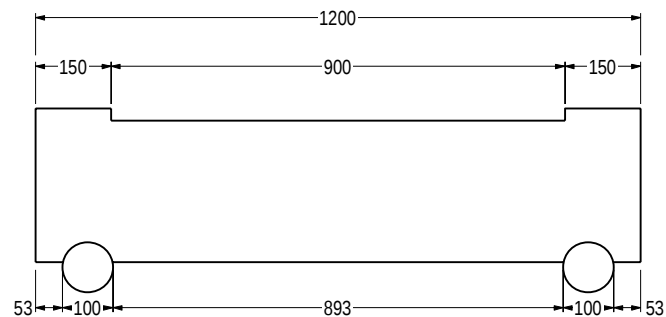
VISTA EN ALZADO Escala: 1:15
