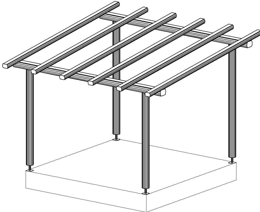
VISTA EN AXONOMÉTRICA Escala: 1:10
